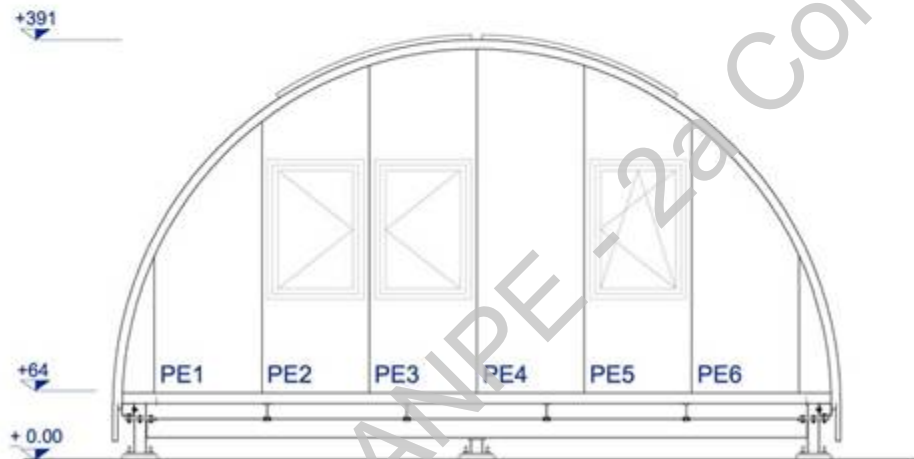
PROSPETTI - scala 1:50
