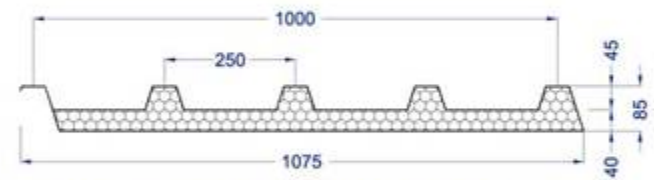
PANNELLI ELYCOP CON FINITURA METALLICA FISSATI ALLA STRUTTURA PORTANTE CON VITI AUTOFIETTANTI scala 1:50
