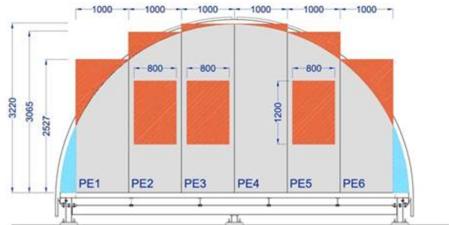
ABACO PANNELLI ESTERNI CON INDICAZIONE SFRIDI - scala 1:50
