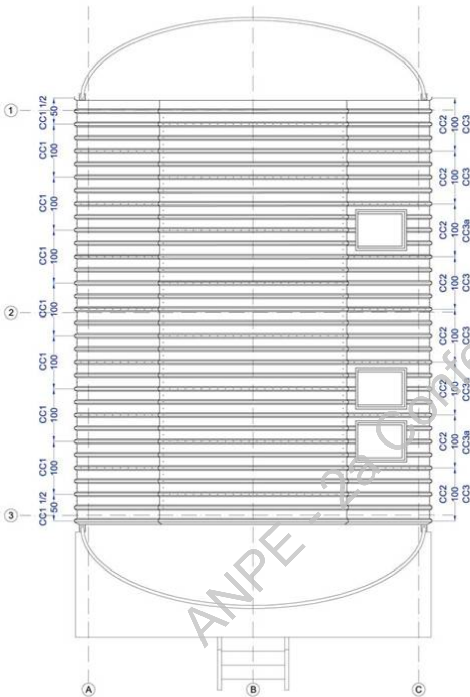
PANNELLI ELYCOP CON FINITURA METALLICA FISSATI ALLA STRUTTURA PORTANTE CON VITI AUTOFIETTANTI scala 1:50
